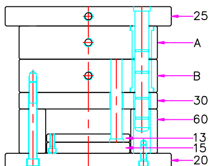
GAI
