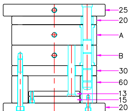
FAI
